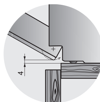
Detail Y
