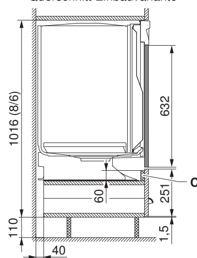
Querschnitt Einbauvariante
