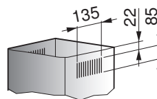
Luftsaustritt bei Umluft (Detail Y)
