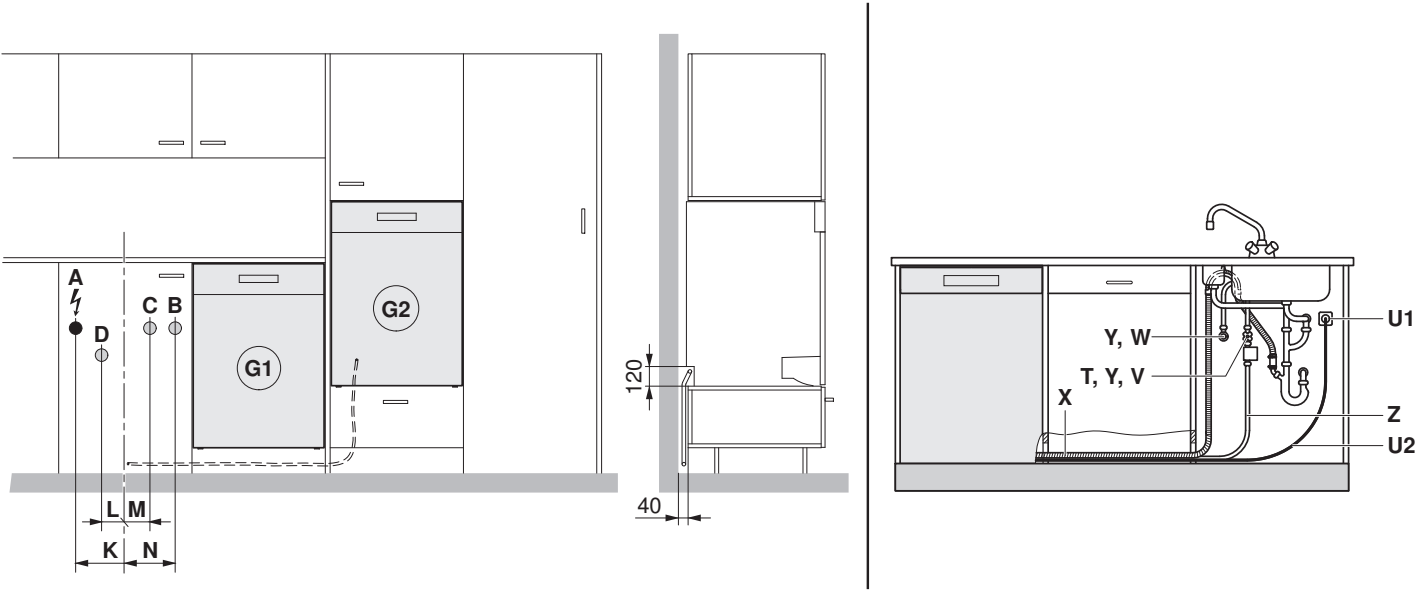
Anschlussbeispiel
